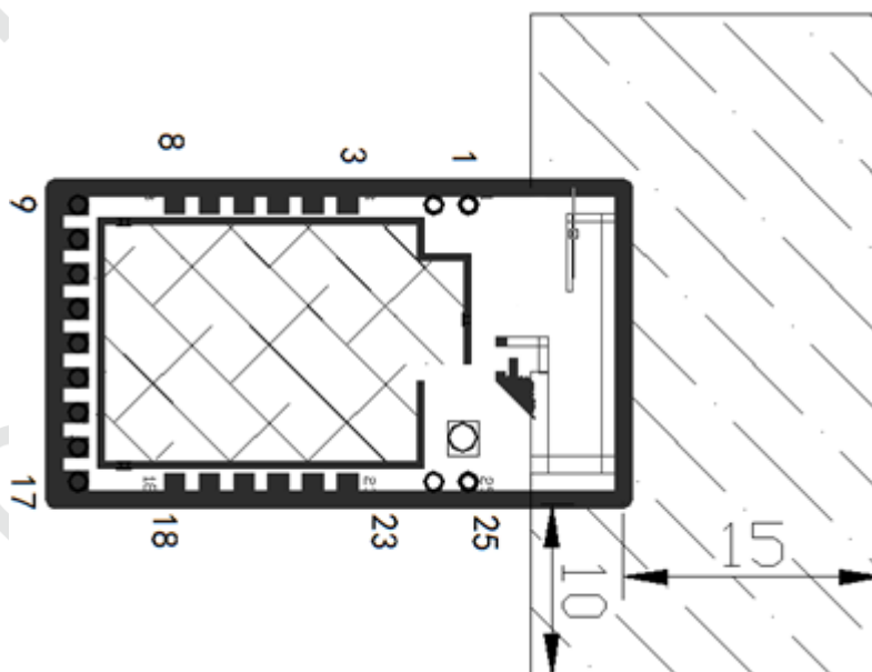
图 2.10 PCB 天线最小净空区
