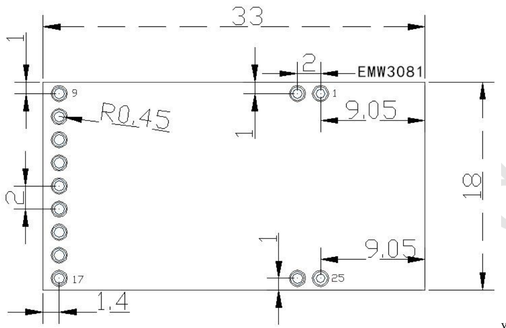
图 2.3DIP 封装
