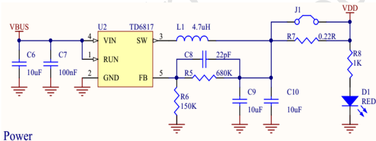
图 2.5 电源转换部分
