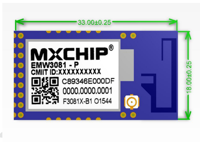
图 2.1 机械尺寸俯视图
