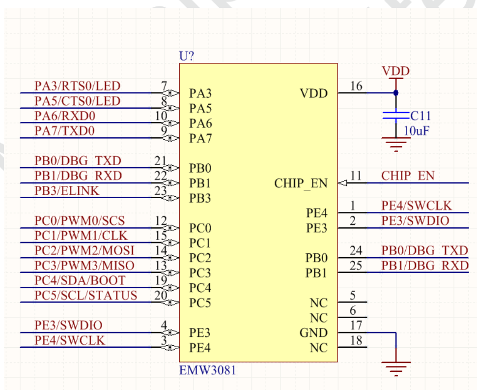
图 2.8 Wi-Fi 参考设计电路
