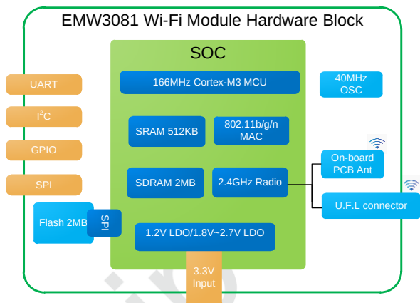
图 1.2 硬件框图
