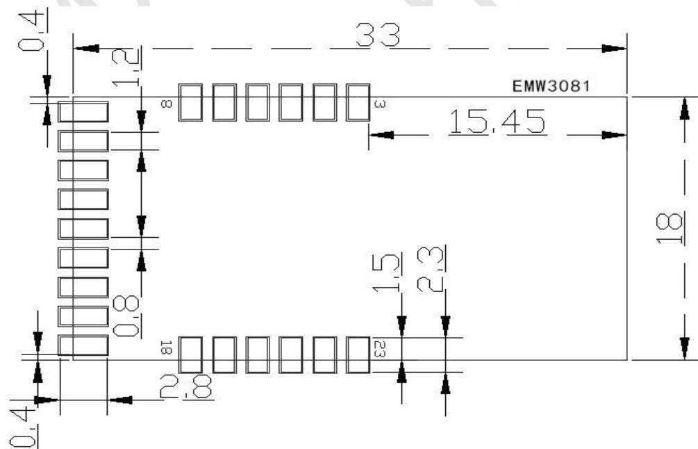
图 2.4 SMT 推荐封装
