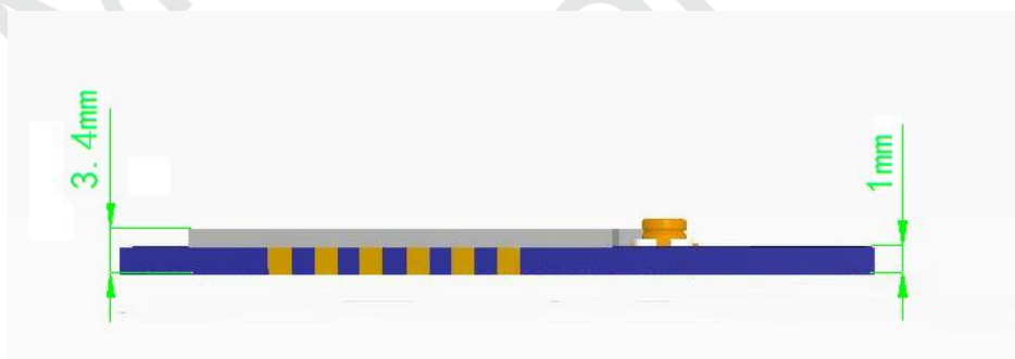
图 2.2 机械尺寸侧视图
