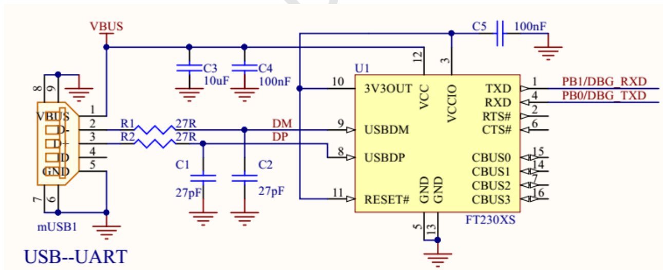
图 2.6 USB 转串口调试参考电路
