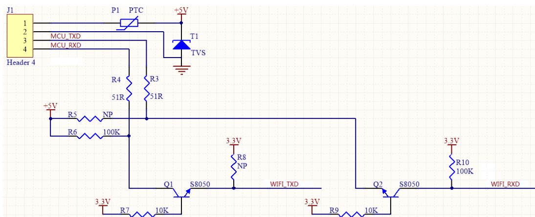
图 2.7 5V UART 转 3.3V UART 转换参考电路
